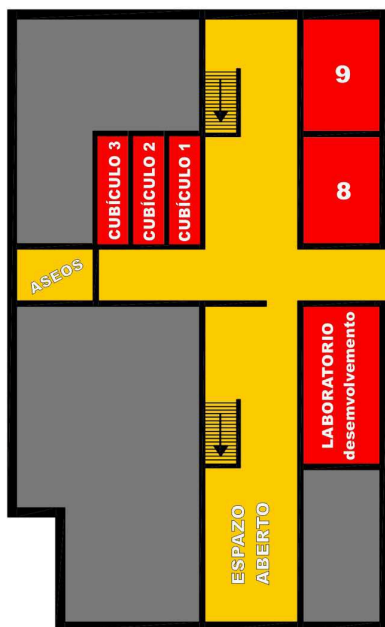
PLANTA BAIXA
