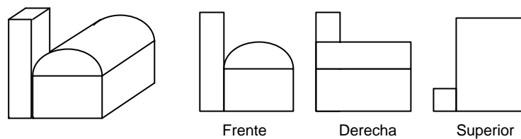
Figura 20. Dibujo de las proyecciones ortogonales de un edificio.
