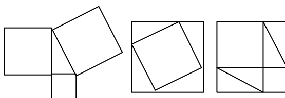
Figura 16. Demostración visual del teorema de Pitágoras
