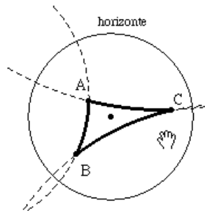
Figura 15. Un triángulo hiperbólico en el disco de Poincaré.
